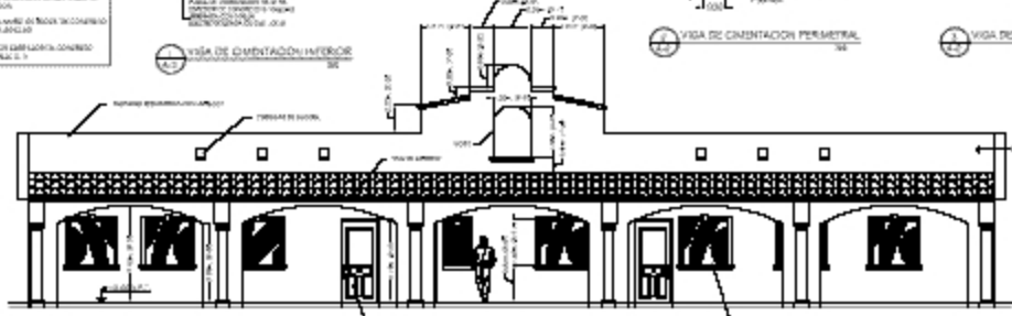
ELEVACIÓN FRONTAL 001
