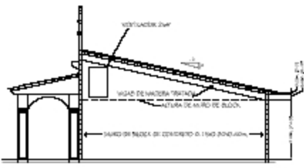
ELEVACIÓN LATERAL 001
