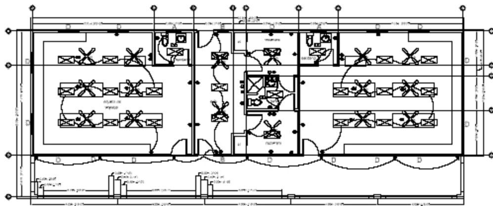
PLANTA ARQUITECTÓNICA 100
